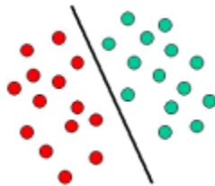
Linear Classifier
